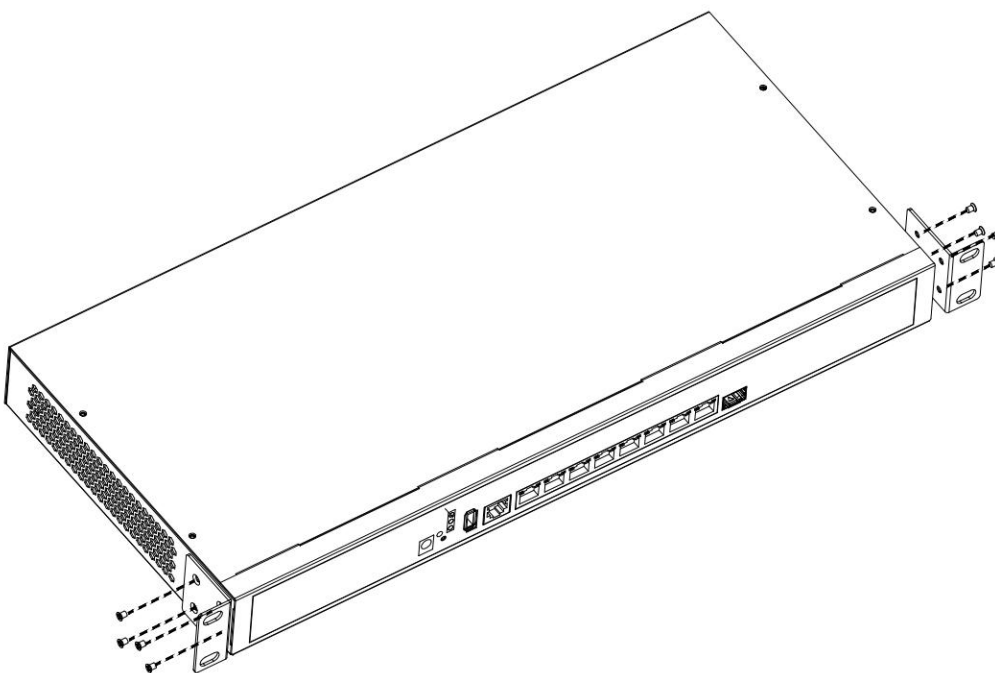
图2-1 将角铁固定在网关上
