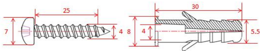
图 1-4 XMG-3200 壁挂安装螺丝尺寸图（单位 mm）
