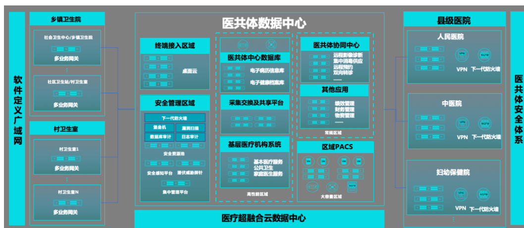
医共体基础网络架构解决方案拓扑
