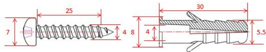
图 1-4 SFG-2520-PWR 壁挂安装螺丝尺寸图（单位 mm）
