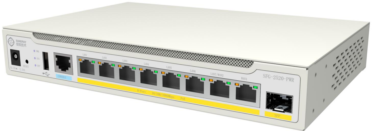
图 1-1 信锐 SFG-2520-PWR 正面图
