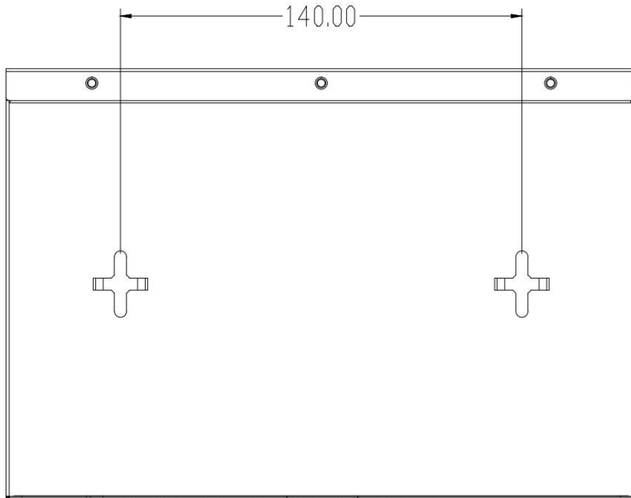
图 1-3 SFG-2520-PWR 尺寸图
