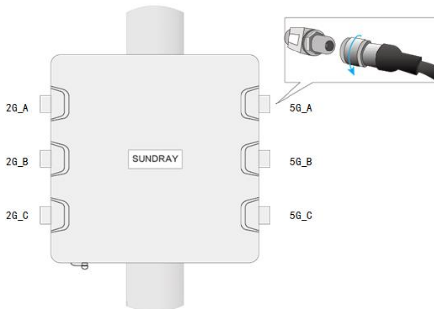
图 3-11 连接馈线示意图
