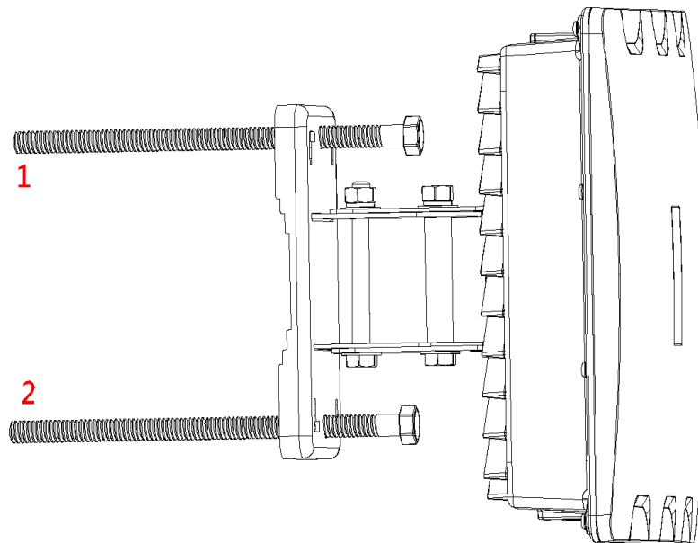
图 3-4 穿螺丝示意图
