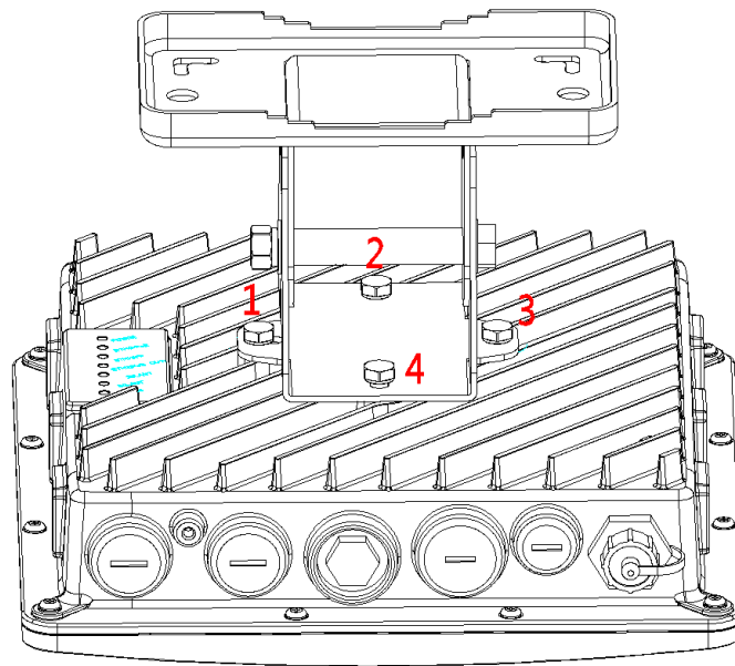
图 3-3 安装主抱杆示意图
