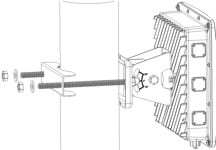
图 3-6 将 AP 固定到抱杆上示意图
