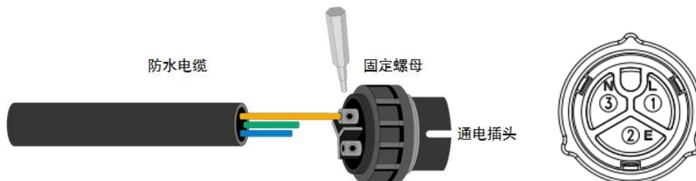
图 3-17 接电线到插头
