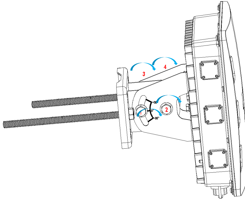
图 3-5 调整 AP 角度示意图
