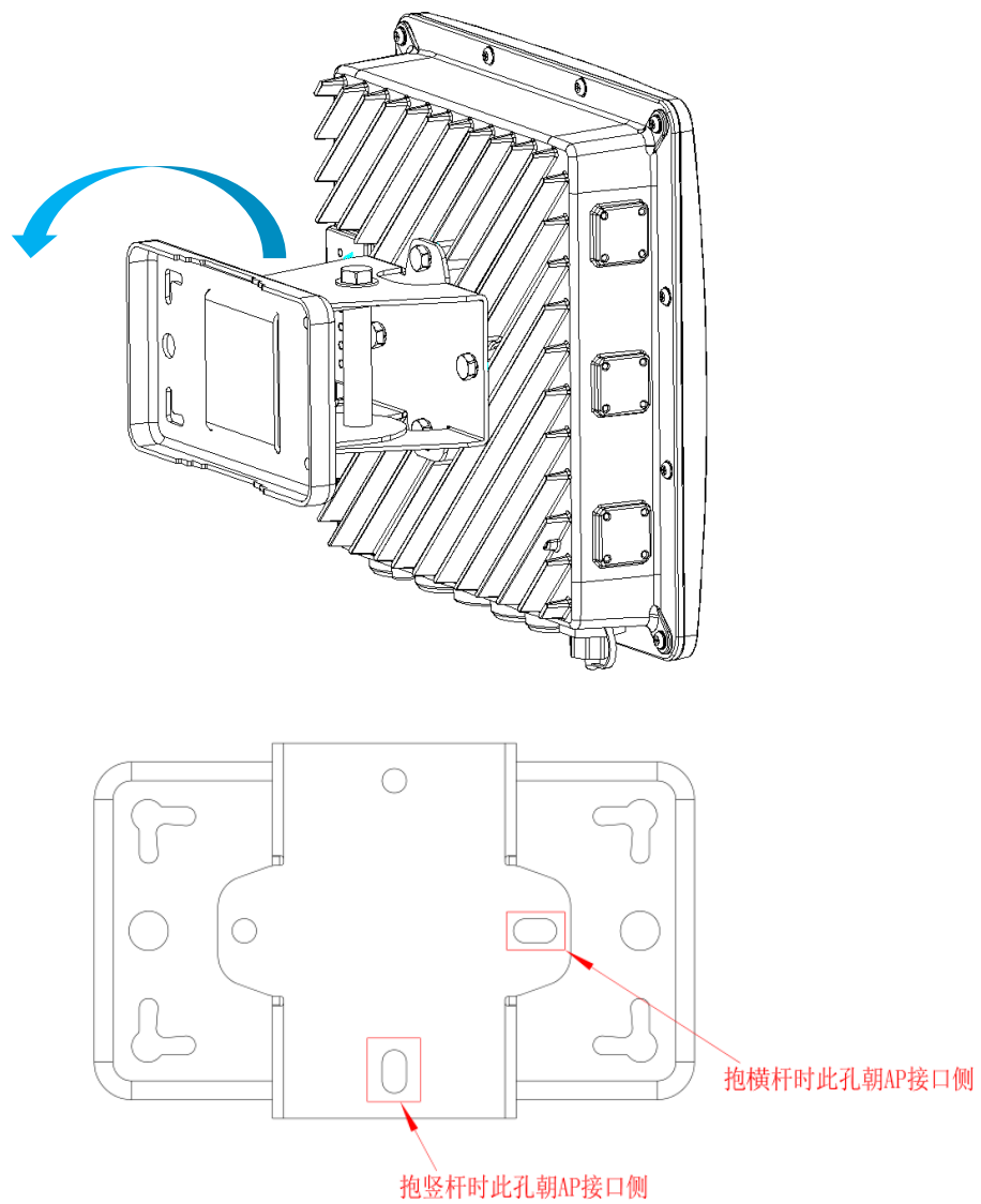
图 3-7 抱横杆安装示意图
