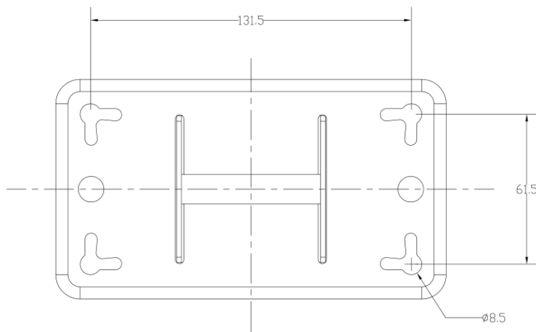
图 3-1 支架 1 正视抱杆尺寸
