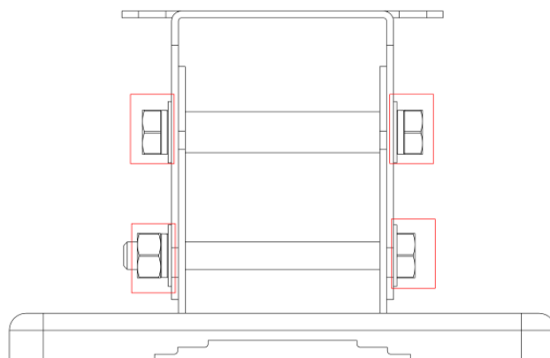
图 3-2 支架俯视图
