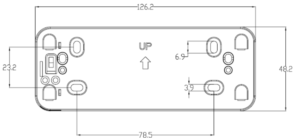
图 3-1 AP-MountKit-T4 支架尺寸图（单位 mm）
