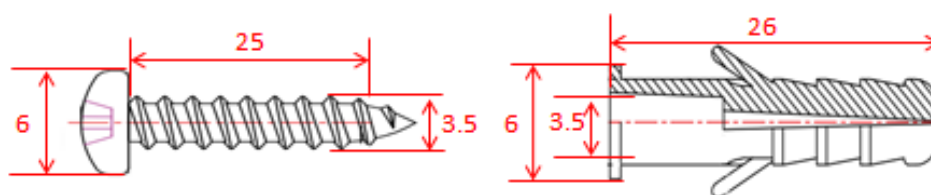
图 3-2 AP-MountKit-T4 壁挂安装螺丝尺寸图（单位 mm）
