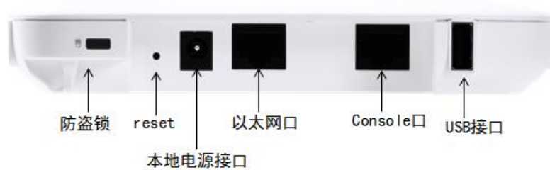
图 1-2 产品侧面接口图
