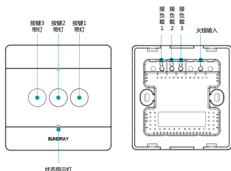
信锐 3 路智能触摸单火开关 SI-SW-M3-T3-Z
