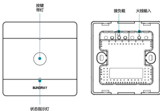
信锐 1 路智能触摸单火开关 SI-SW-M3-T1-Z
