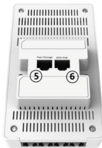
1-2 产品背面图
