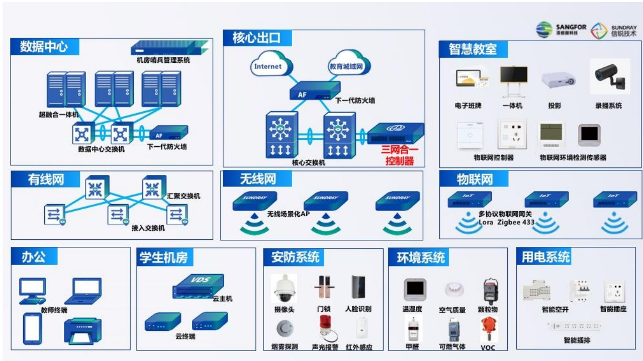
智慧校园 IT 基础设施架构图
