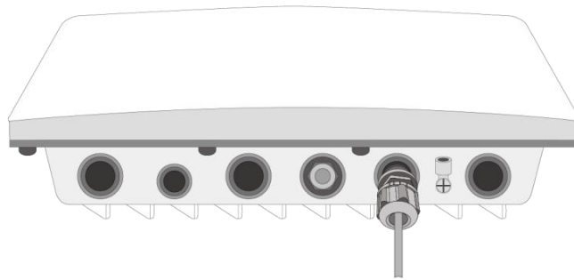
图 3-12 连接网线示意图二
