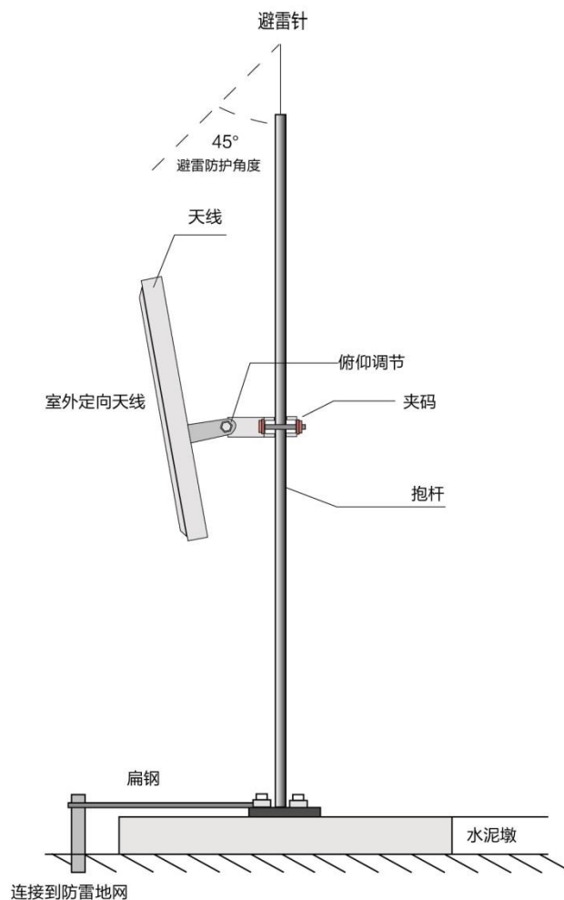
图 3-9 定向天线安装示意图
