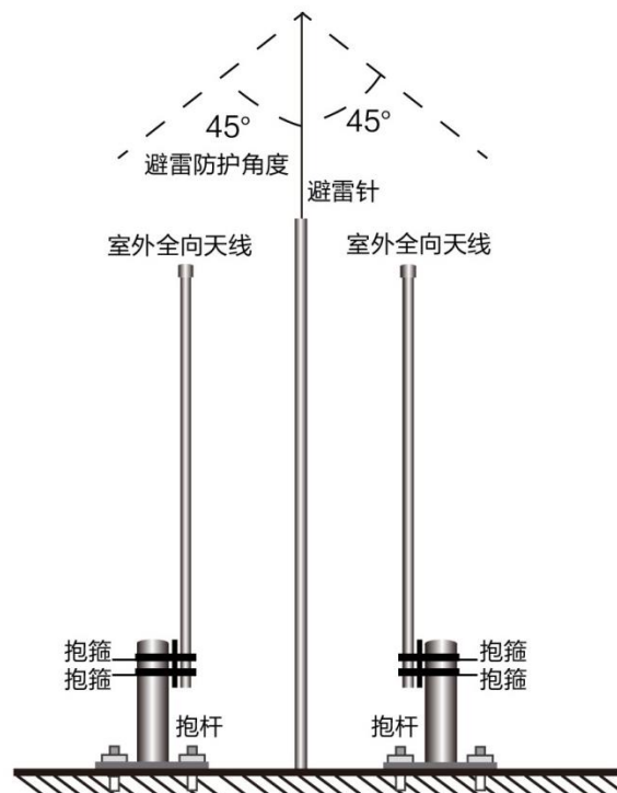
图 3-8 全向天线安装示意图
