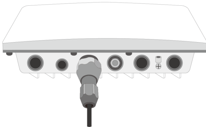
图 3-14 连接光纤示意图二
