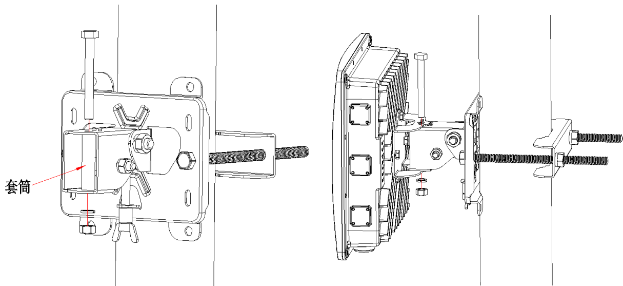
图 3-5 将 AP 固定到抱杆上示意图
