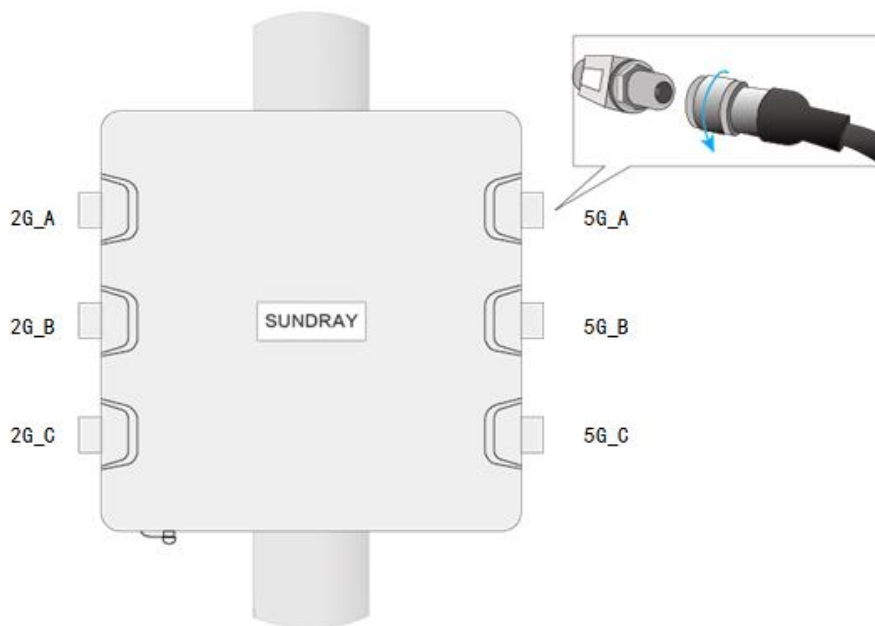
图 3-10 连接馈线示意图
