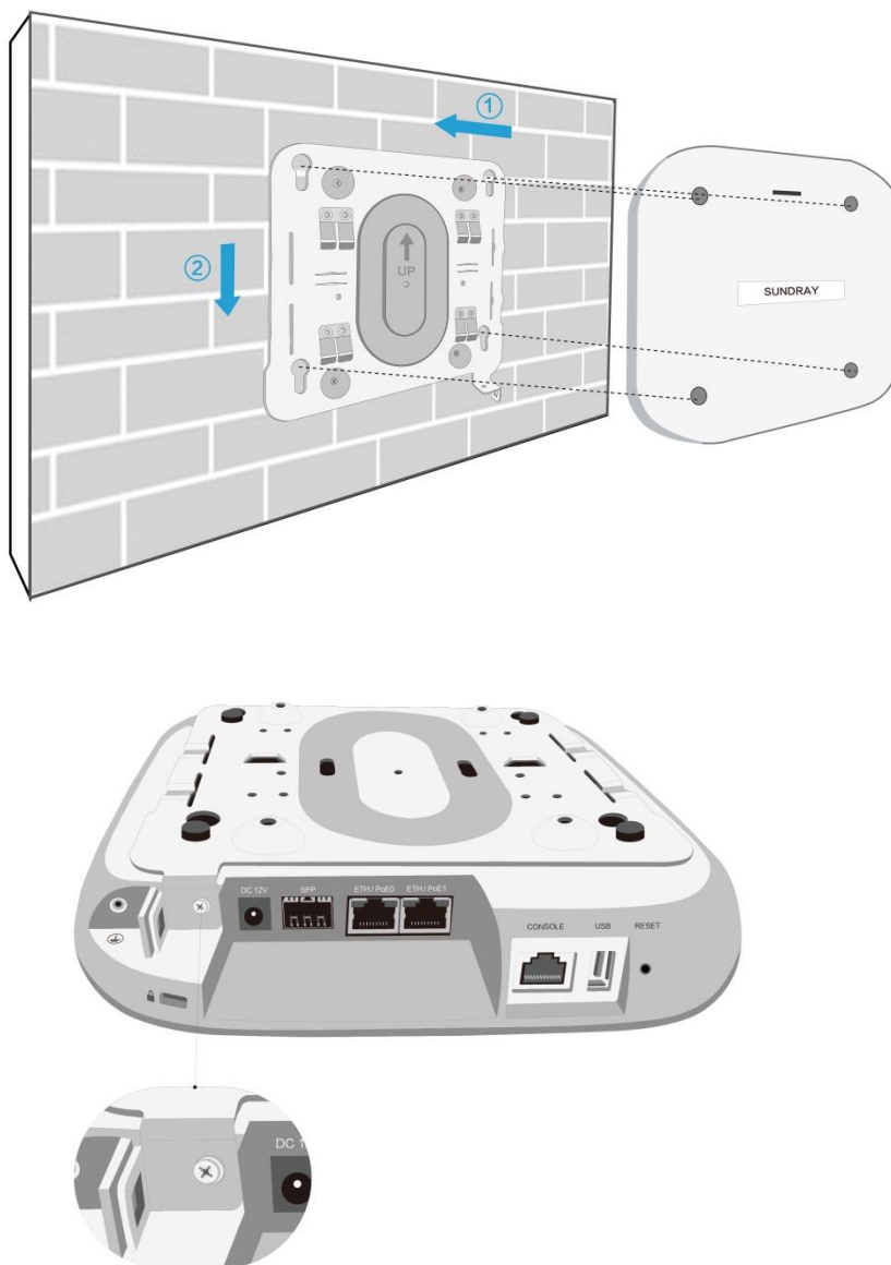
图 3-6 AP 安装到壁挂支架示意图
