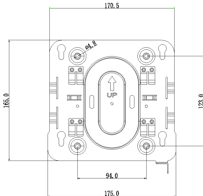
图 3-1 NAP-5600 支架尺寸图（单位 mm）
