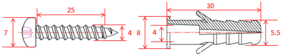
图 3-2 NAP-5600 壁挂安装螺丝尺寸图 (单位 mm)
