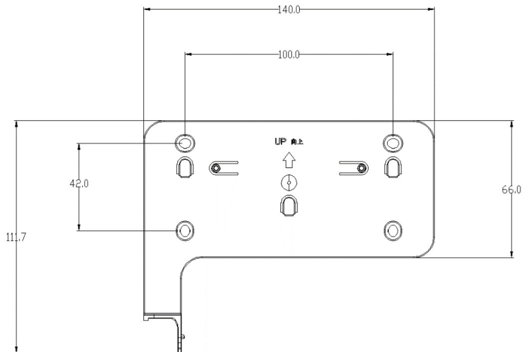
图 3-1 NAP-3700 支架尺寸图（单位 mm）
