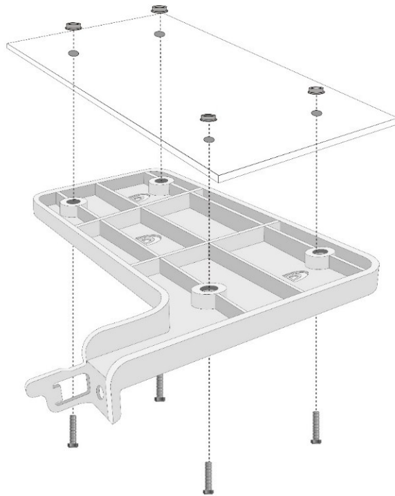
图 3-8 吸顶支架安装示意图
