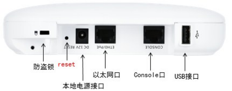
图 1-2 产品侧面接口图
