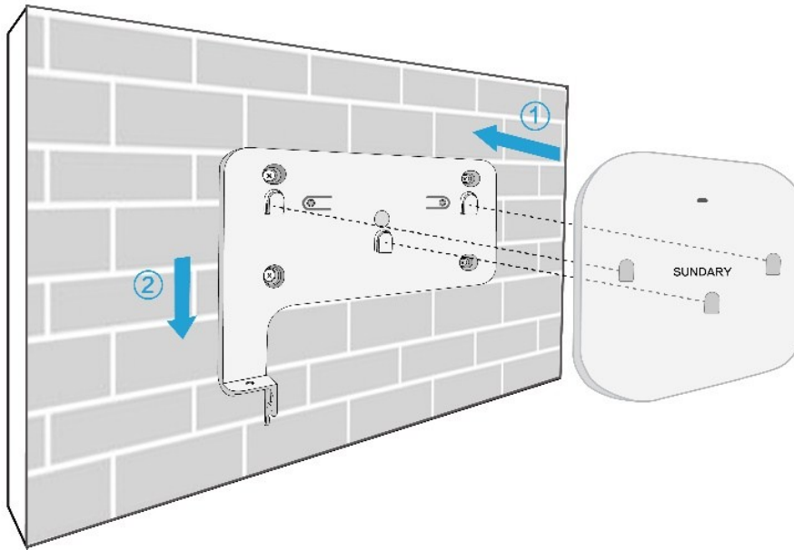
图 3-6 AP 安装到壁挂支架示意图
