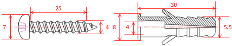
图 3-2 NAP-3700 壁挂安装螺丝尺寸图 (单位 mm)
