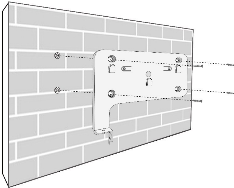
图 3-5 壁挂支架安装示意图
